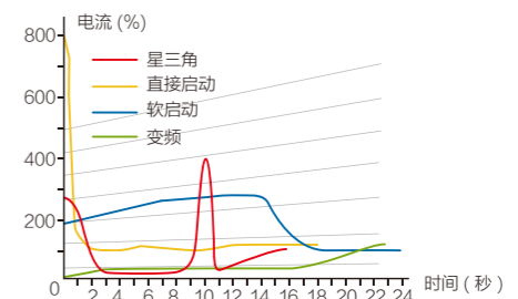
启动电流表
