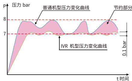
压力变化图
