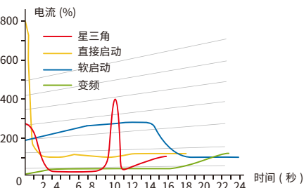
启动电流表
